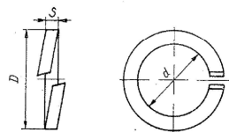
ШАЙБА ПРУЖИННАЯ SPRING WASHER GLATTE FEDERRING RONDELLE ELASTIQUE ARANDELA DE RESORTE
