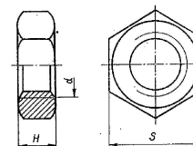
ГАЙКА ШЕСТИГРАННАЯ НИЗКАЯ LOW HEXAGON NUT SECHSKANTFLACHMUTTER ECROU A SIX PANS A REBORD BAS TUERCA BAJA DE SEIS ARISTAS
