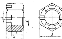
ГАЙКА ШЕСТИГРАННАЯ ПРОРЕЗНАЯ SLIT HEXAGON NUT SECHSKANTSCHLITZMUTTER ECROU A SIX PANS A ENTAILLES TUERCA DE SEIS ARISTAS RANURADA
