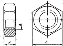
ГАЙКА ШЕСТИГРАННАЯ НИЗКАЯ LOW HEXAGON NUT SECHSKANTMUTTER ECROU A SIX PANS TUERCA DE SEIS ARISTAS
